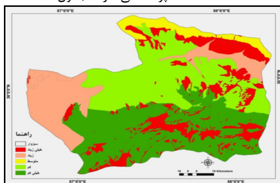
نقشه ۱۲- کلاسه‌بندی خطر سیل خیزی در شهرستان سبزوار (مآخذ: نویسندگان، ۱۳۹۹)
