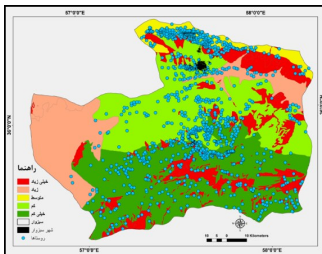
نقشه ۱۳- نهایی کلاسه‌بندی خطر سیل خیزی در شهرستان سبزوار (مآخذ: نویسندگان، ۱۳۹۹)
