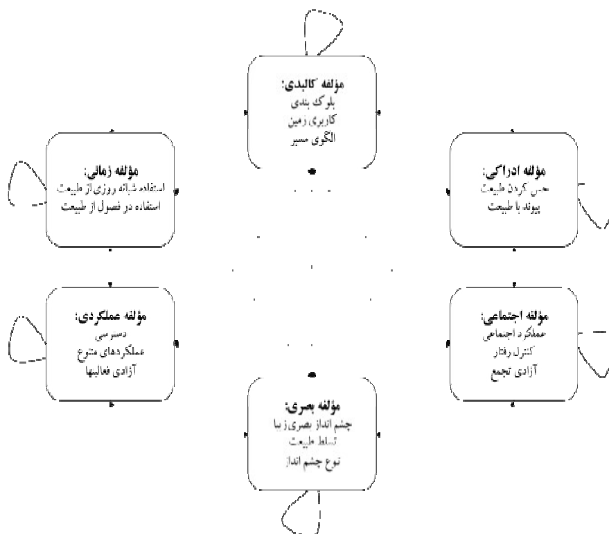
شکل ۸- مدل شبکه‌ای ANP برای شاخص‌های سرزندگی
